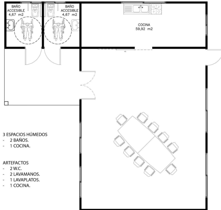
Planta de Arquitectura Proyecto FRIL 2025 “Construcción Sede Comunitaria Villa Santa María, Catemu”. Fuente Cargada Proyecto FRIL.
